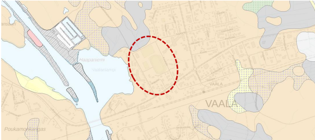
Alueen maaperä. Oranssilla värillä on esitetty hiekkamoreeni, violetilla saraturve. (Kartta maaperä 1:20 000 GTK Maankamara).
